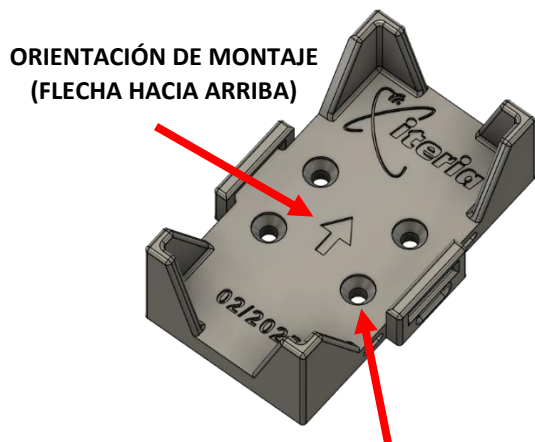
ORIFICIOS PARA TORNILLOS DE FIJACIÓN M4 AVELLANADOS
