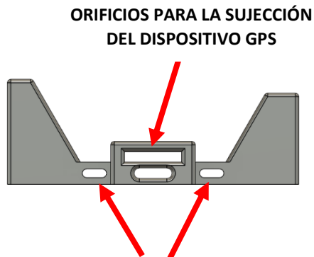
ORIFICIOS PARA SUJECCIÓN CON BRIDAS AL VEHÍCULO
